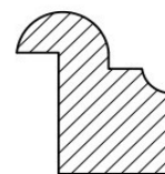
201-G 18 x 20 mm. rebajo 15 x 5 mm.
